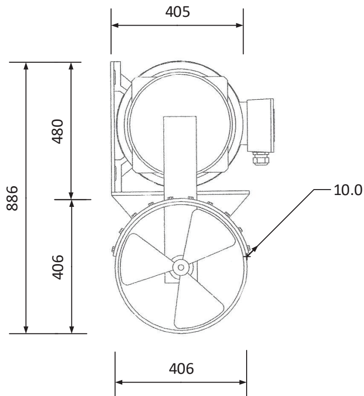
Vooraanzicht
